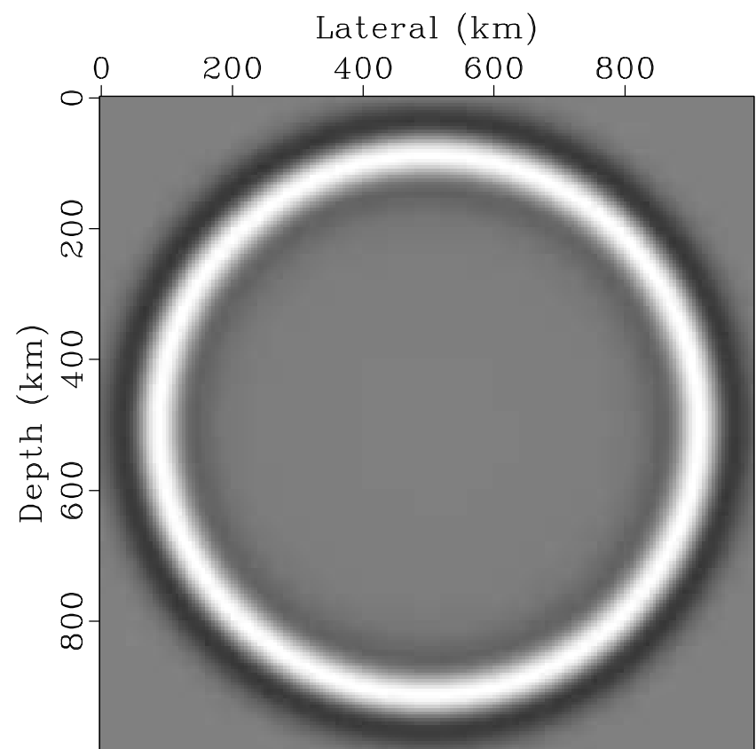
Backward: t=0.28\text{s}
