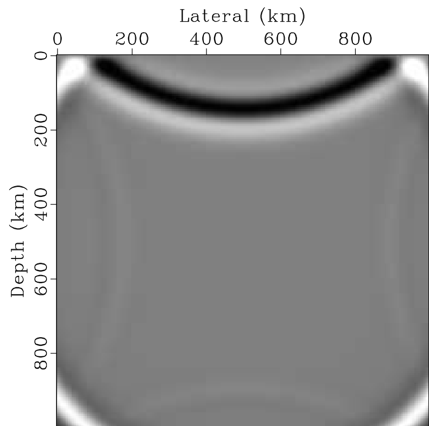
Backward: t=0.4\text{s}
