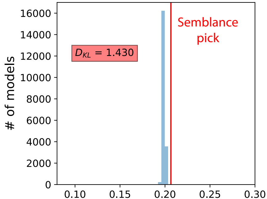
Posterior for W
