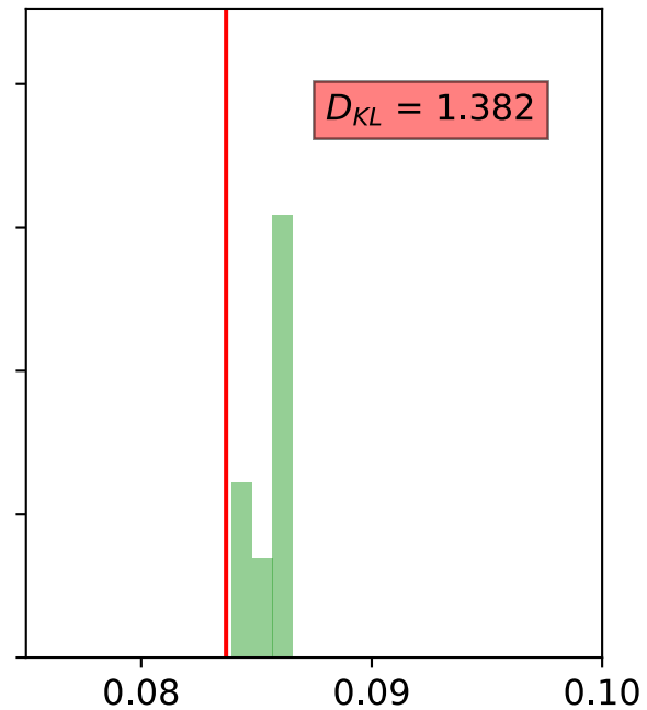
Posterior for W_3
