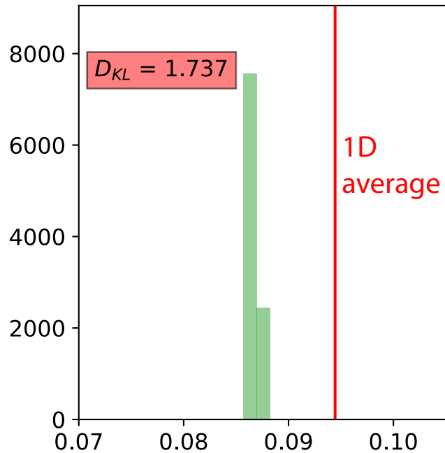
Posterior for W_1
