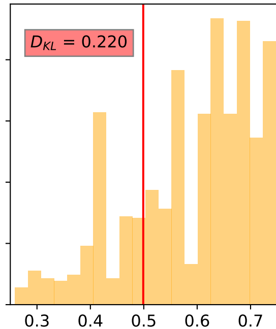
Posterior for B_3
