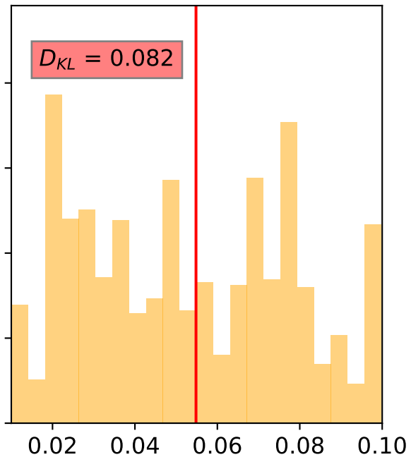
Posterior for B_2
