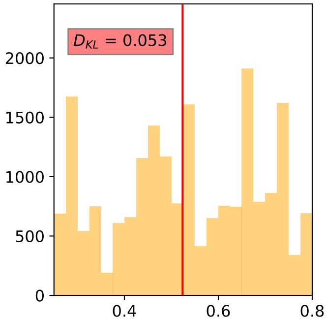
Posterior for B_1
