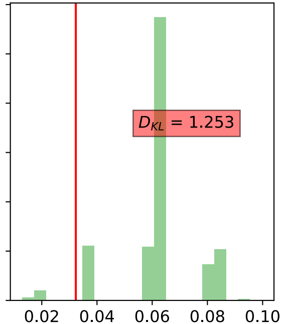
Posterior for B_2
