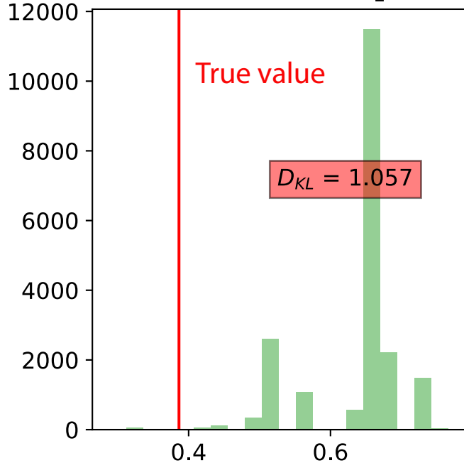
Posterior for B_1
