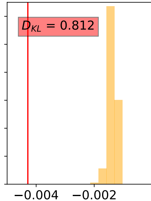
Posterior for A_3
