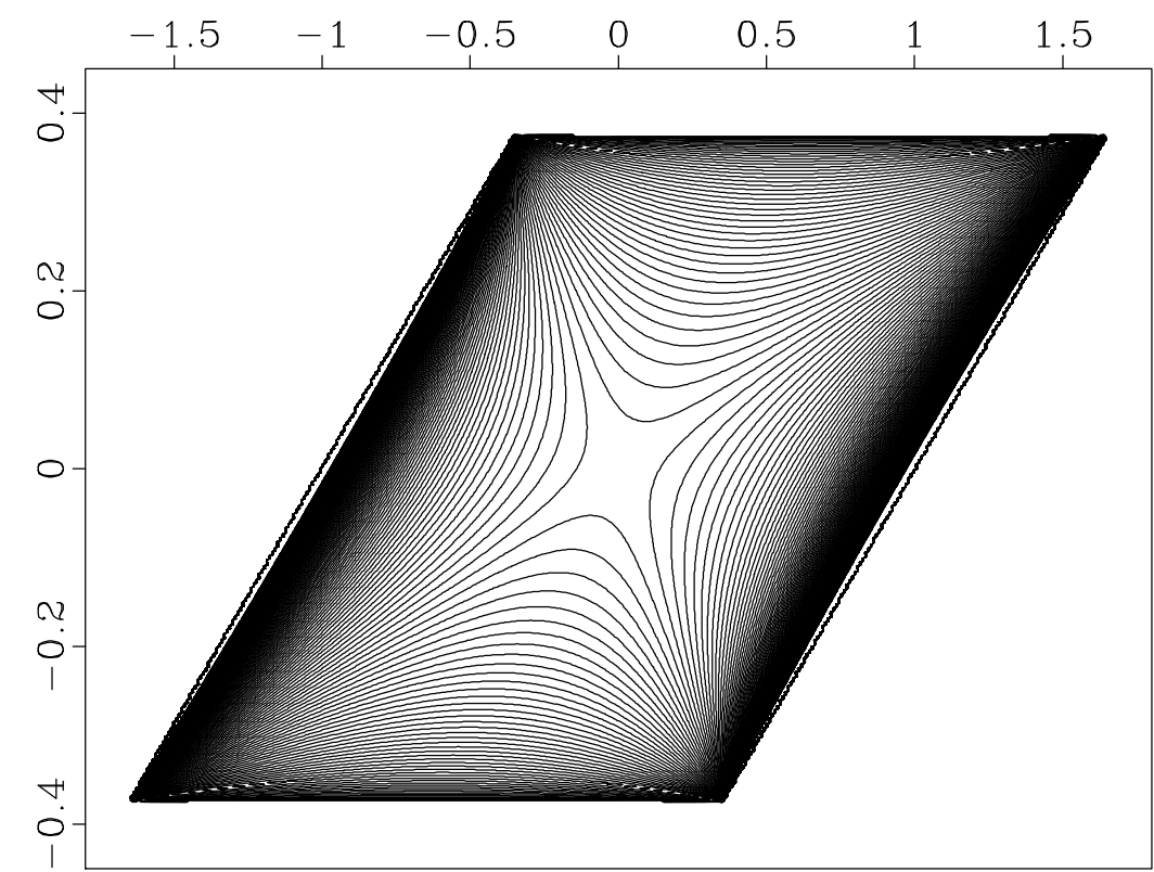
AMO impulse response: \phi=30 , v=10 m/s
