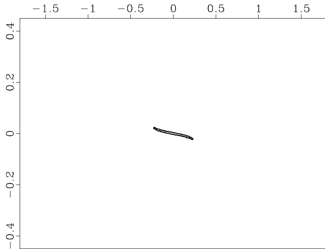
AMO impulse response: \phi=3 , v=2000 m/s
