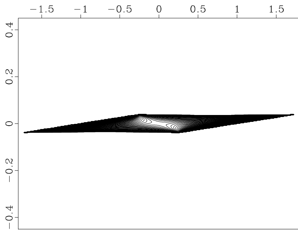
AMO impulse response: \phi=3 , v=10 m/s
