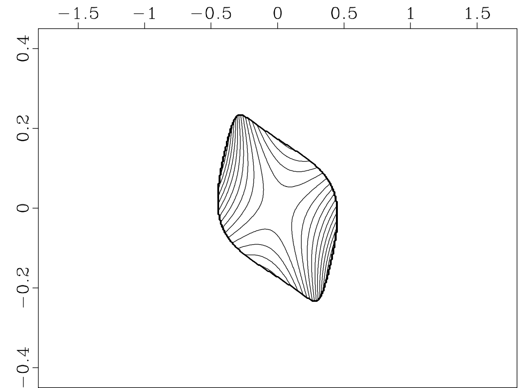
AMO impulse response: \phi=30 , v=2000 m/s
