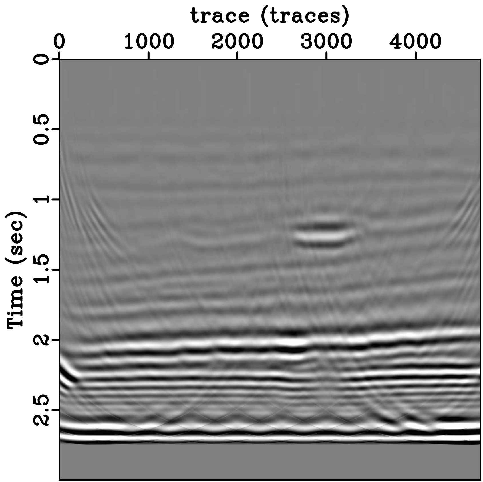
Kirchhoff Post Stack Mig
